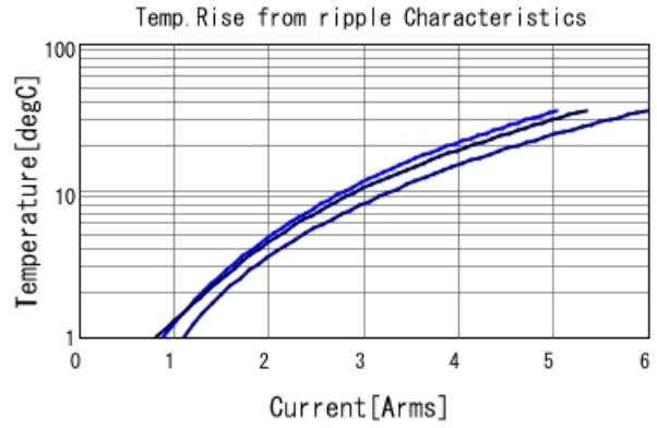
GRT31CC81A106ME01 Temp. rise — 100kHz — 500
