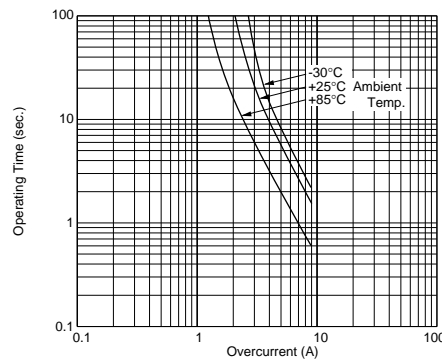
PTGLCSAR0R2M1B51B0
