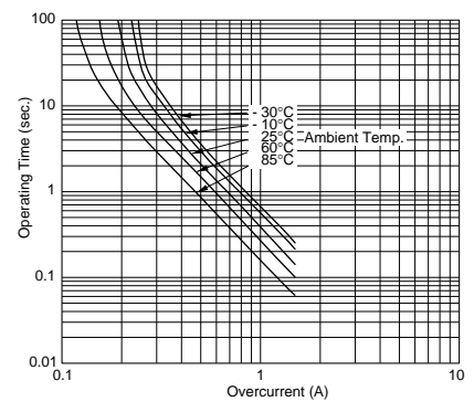
PTGL4SAS100K2N51B0
