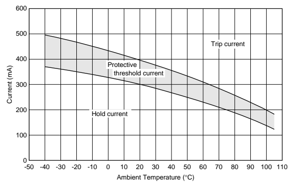
PTGL7SAS5R6K4B51B0
