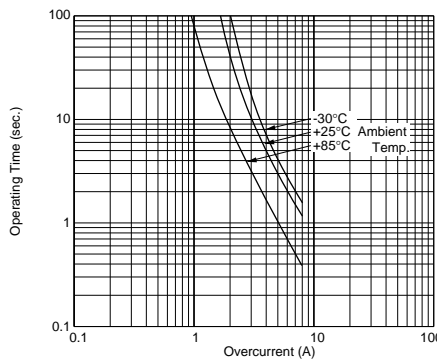
PTGLASARR27M1B51B0
