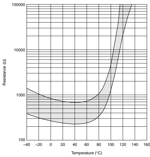
PRF18BC471QS5RB
