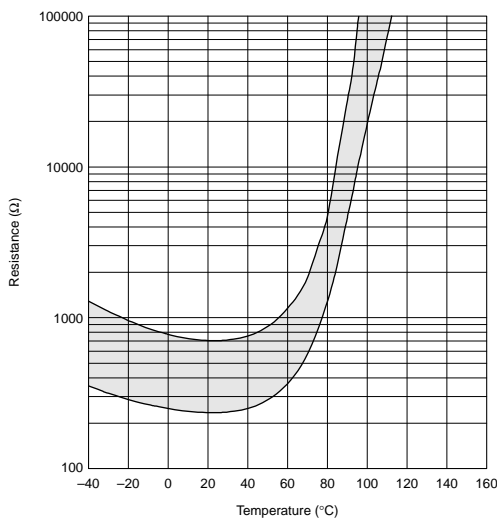
PRF18BE471QS5RB
