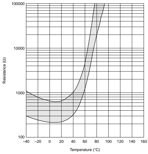
PRF18BG471QS5RB
