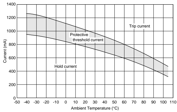
PTGLCSAS1R2K3B51B0
