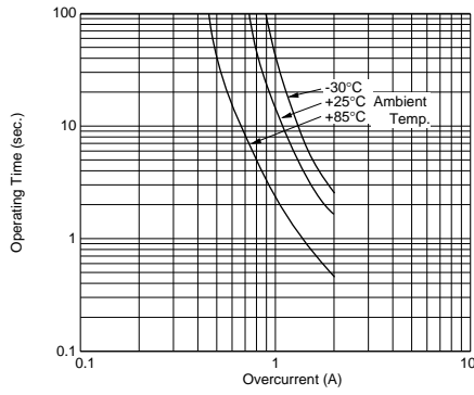
PTGL5SAR1R0M1B51B0
