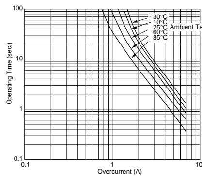
PTGLCSAS0R8K2B51B0
