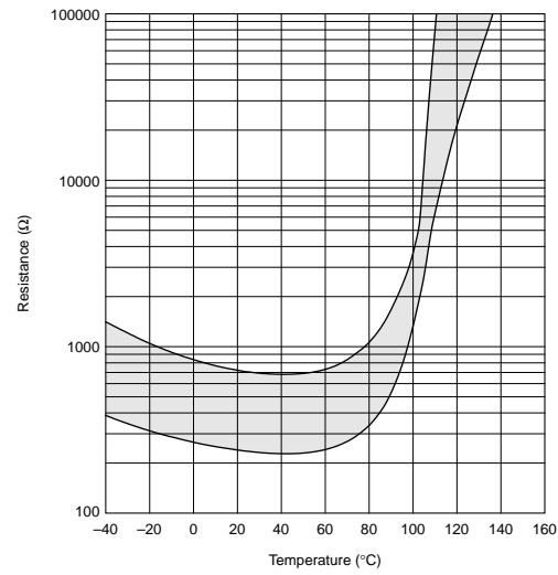
PRF18BC471RS5RB
