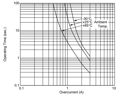
PTGL6SAR0R8M1B51B0
