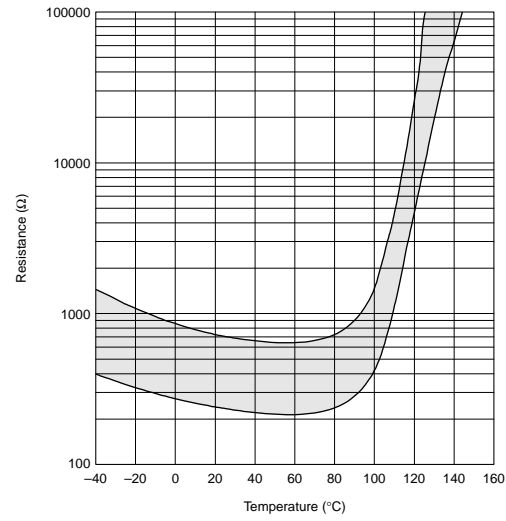
PRF18BB471QS5RB
