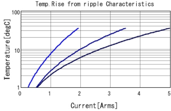
GR355DD72E474KW01 Temp. rise — 30kHz — 100kHz
