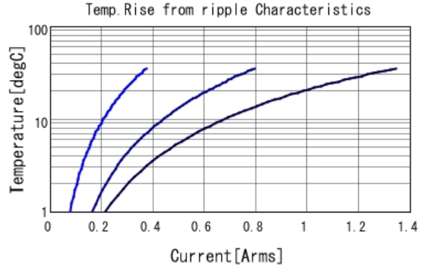
GRJ55DR73A683KWJ1 Temp. rise — 30kHz — 100kHz
