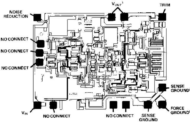
Die Size: 0.081 x 0.060 Inches
