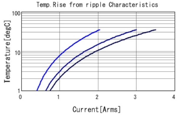
GRM31MR72A474MA35 Temp. rise — 200kHz — 500
