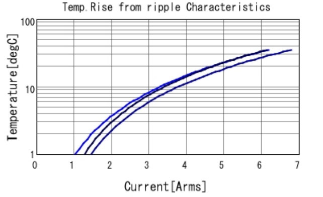
GRM32EE70J476KE20 Temp. rise — 60kHz — 300kHz
