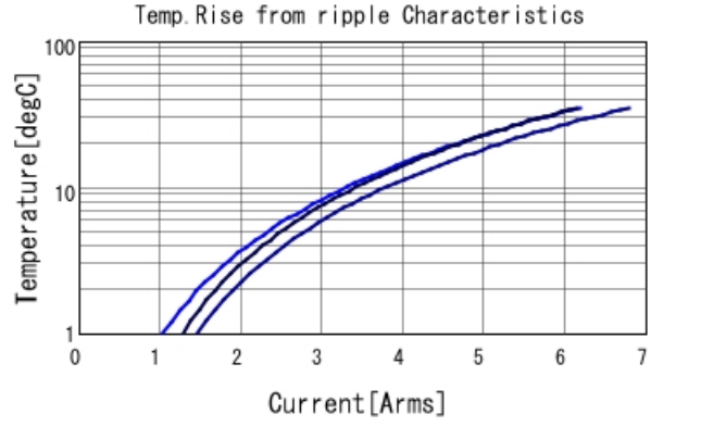
GRM32ED70J476KE20 Temp. rise — 60kHz — 300kHz
