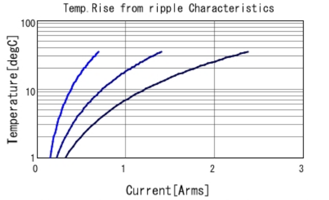
GRJ55DR73A104KWJ1 Temp. rise — 30kHz — 100kHz
