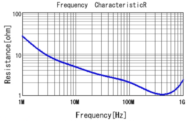
DE2B3SA221KA3BX02F R DCOV, 20degC
