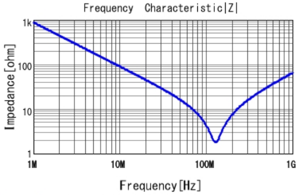
DE2B3SA221KA3BX02F |Z| DCOV, 20degC
