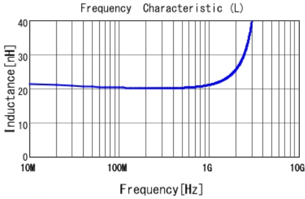
LQW18AN20NJ00 L
