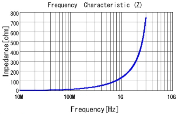
LQW18AN20NJ00 |Z|
