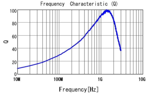
LQW18AN20NJ00 Q
