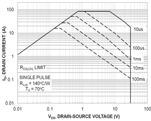
High side FET
