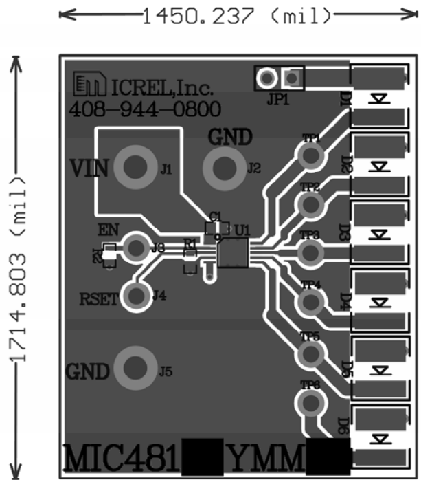
Top Layer
