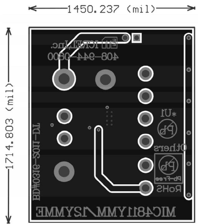
Bottom Layer
